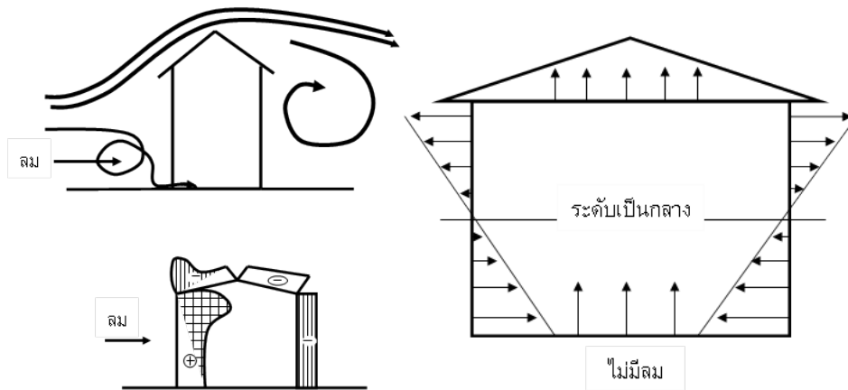
รูปที่ 1 ปัจจัยที่มีผลต่อการรั่วไหลของอากาศเข้าออกอาคารจากลมพัดผ่านอาคารหรืออุณหภูมิภายในและภายนอกที่แตกต่าง (มณีรัตน์ องค์กรบรรณดี, 2556)
