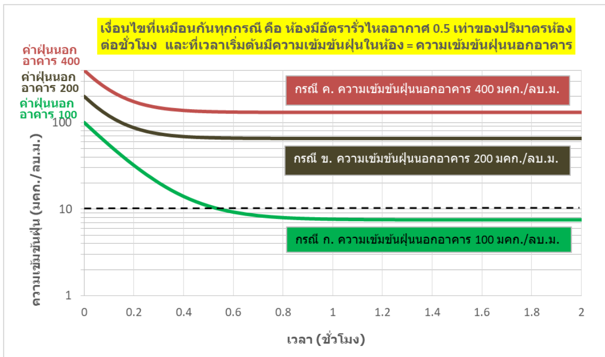
รูปที่ 3 ความเข้มข้นฝุ่นละอองในห้องนอนภายใต้สถานการณ์จำลองที่ 2 ที่มีความเข้มข้นฝุ่นละอองด้านนอกอาคารแตกต่างกัน
